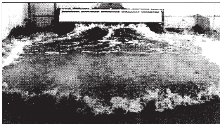
Figura 18: Esempio di sistema di lavaggio di un vaso con un sistema a cacciata.
