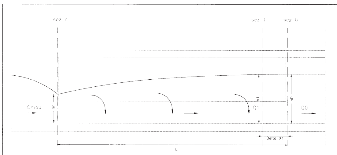
Figura 8: Andamento del pelo libero lungo la soglia dello scolmatore /13/
