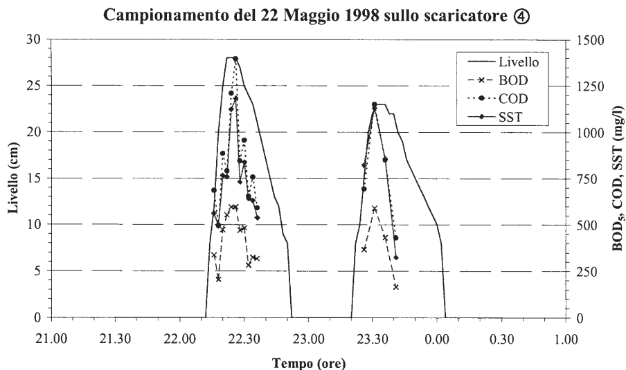
Figura 10: Concentrazione di BOD 5 , COD e SST a valle dello scolmatore
