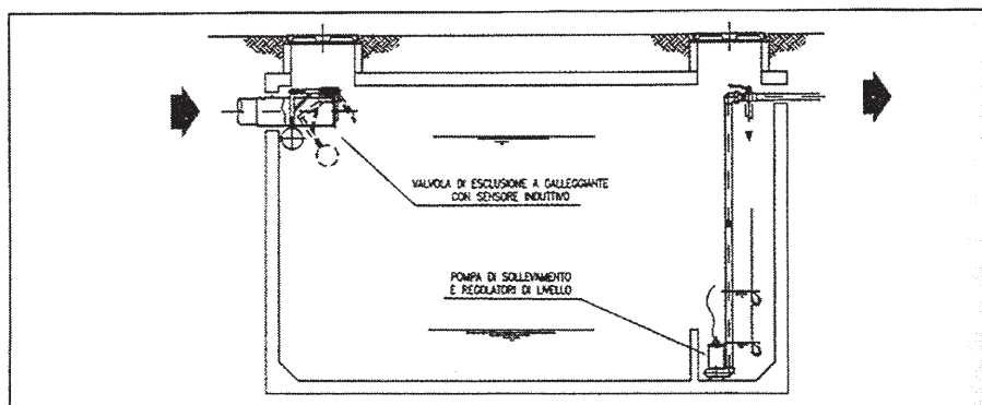
Figura IV.2 Vasca di accumulo: sezione.
