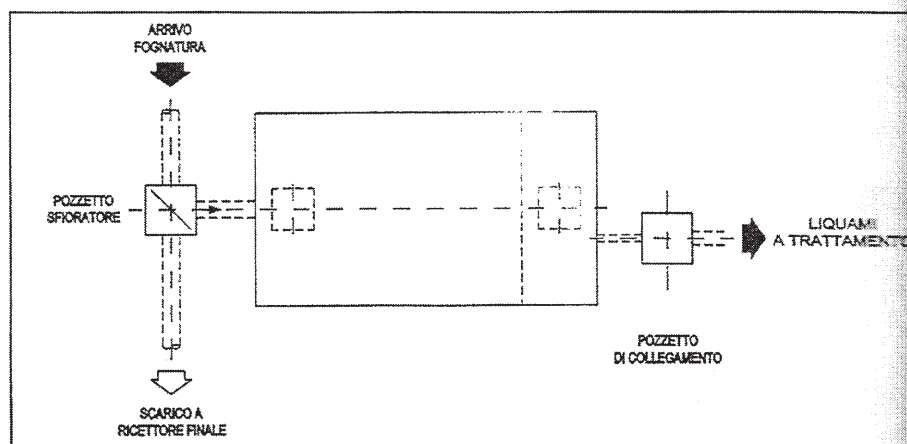
Figure IV.4 Vasca di accumulo: disposizione collega- menti.
