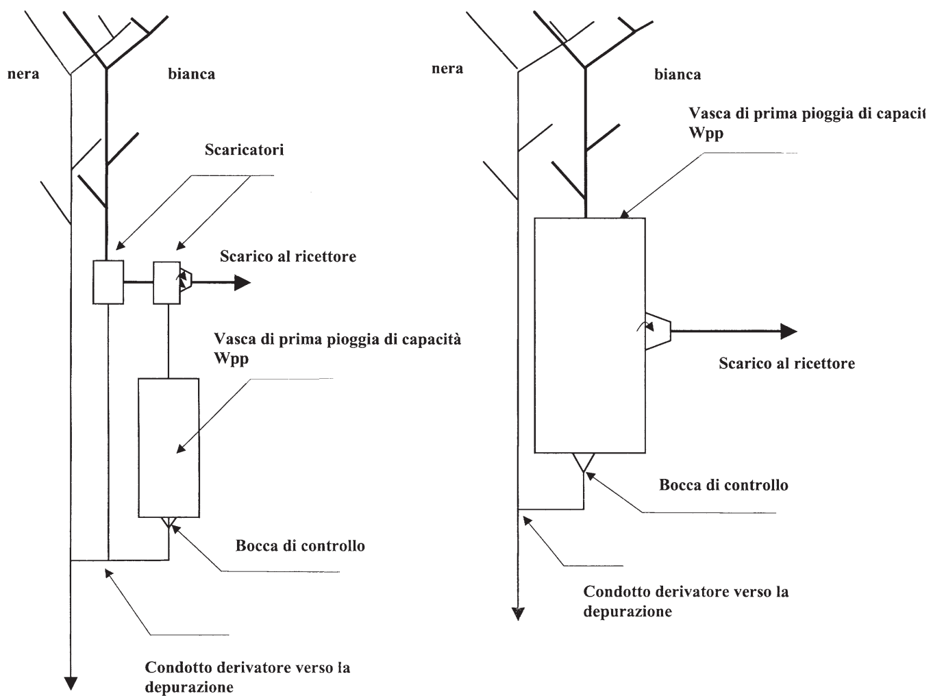
Figura 17: Schemi di reti separate con vasca di prima pioggia, fuori linea o in linea (dove W_{pp} rappresenta il volume di acque di prima pioggia invaso nel nodo) /3/
