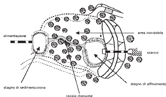
Figura 1 - Schema di un sistema di trattamento Extended Detention Pond
