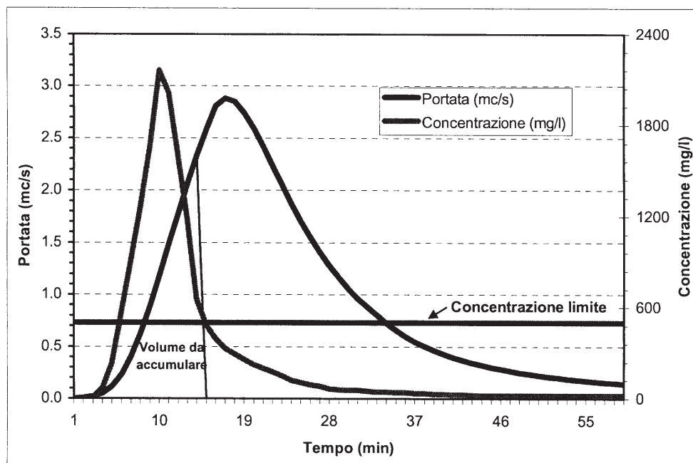
Figura 12: Dimensionamento del volume da assegnare ad una vasca di prima pioggia /6/
