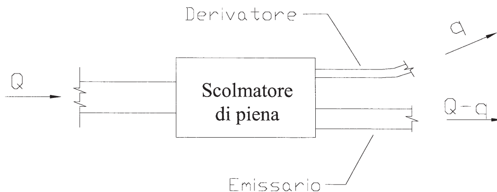
Figura 4: Schema di scolmatore di piena
