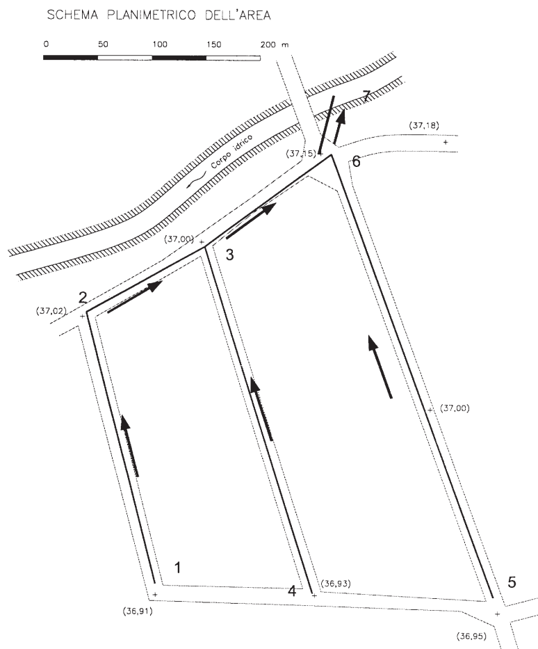
Figura 2: Schema della rete per acque meteoriche
