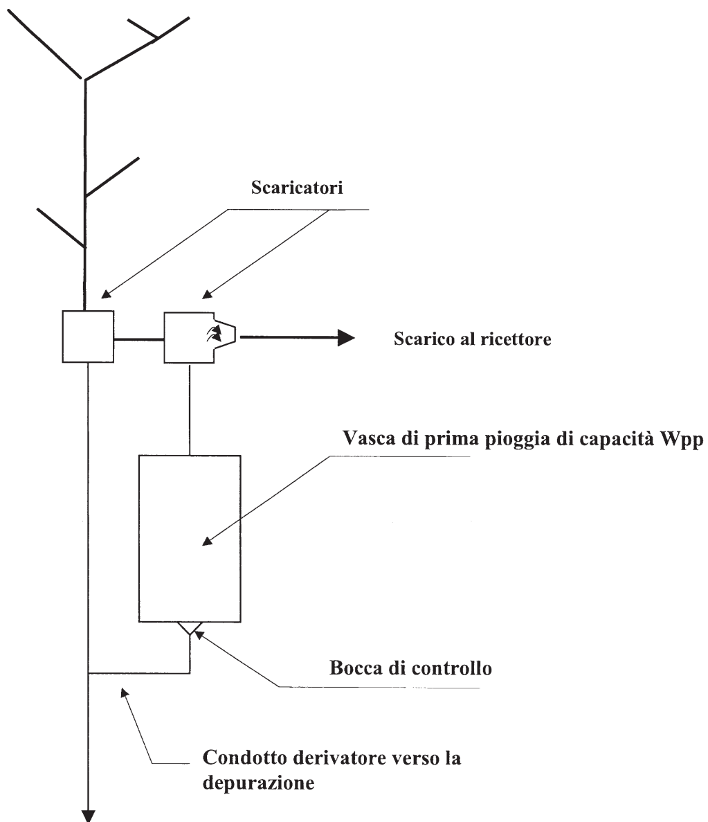
Figura 16: Schemi di reti unitarie con vasca di prima pioggia fuori linea (dove W_{pp} rappresenta il volume di acque di prima pioggia invasato nel nodo) /3/
