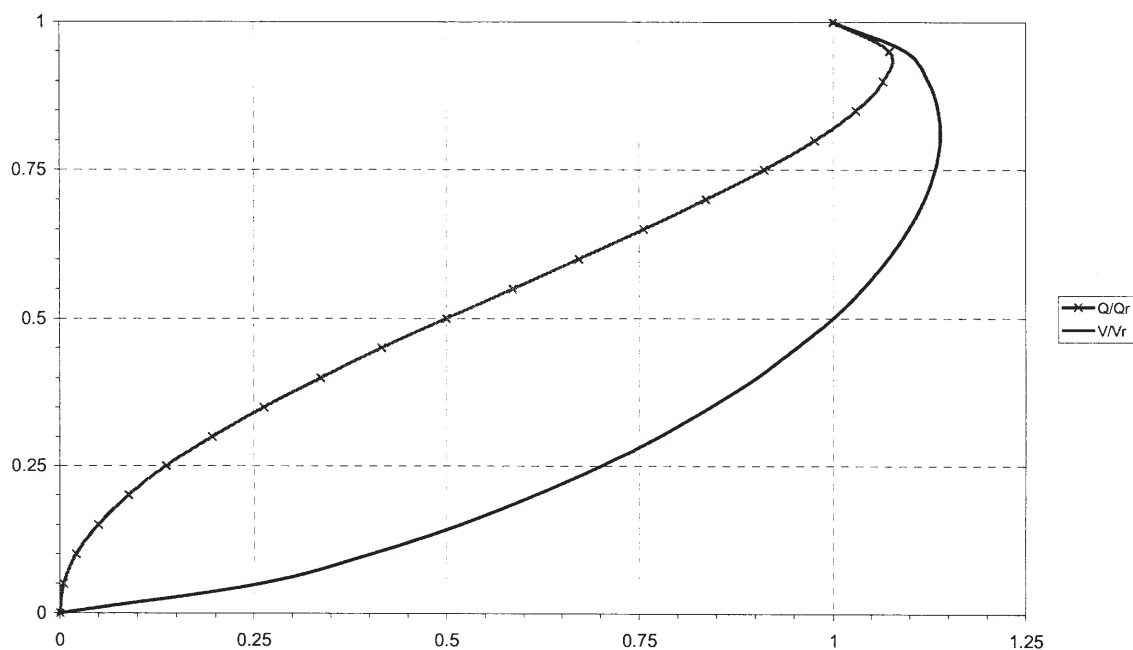
Figura 3: Scala delle portate e delle velocità per sezione circolare.
