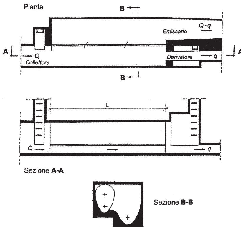
Figura 5: Schema di scolmatore laterale a soglia bassa /3/
