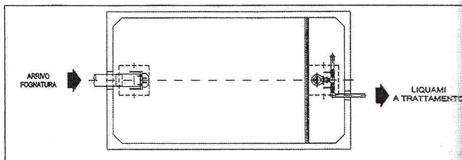
Figura IV.3 Vasca di accumulo: pianta.
