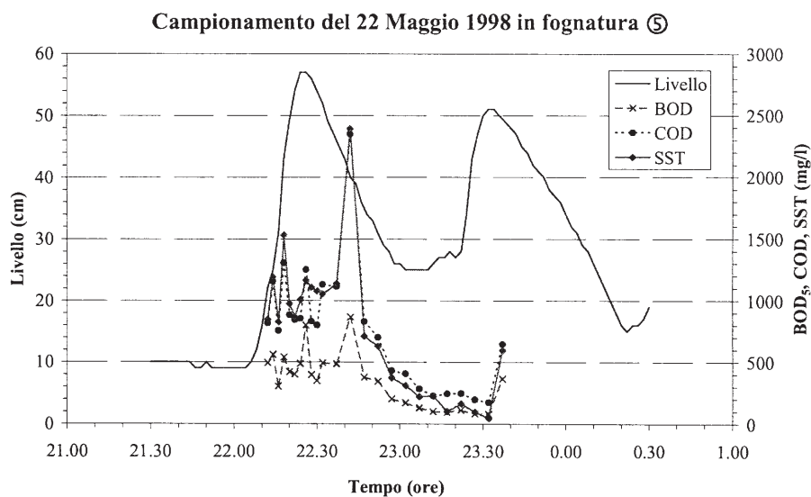
Figura 9: Concentrazione di BOD 5 , COD e SST nel condotto di fognatura
