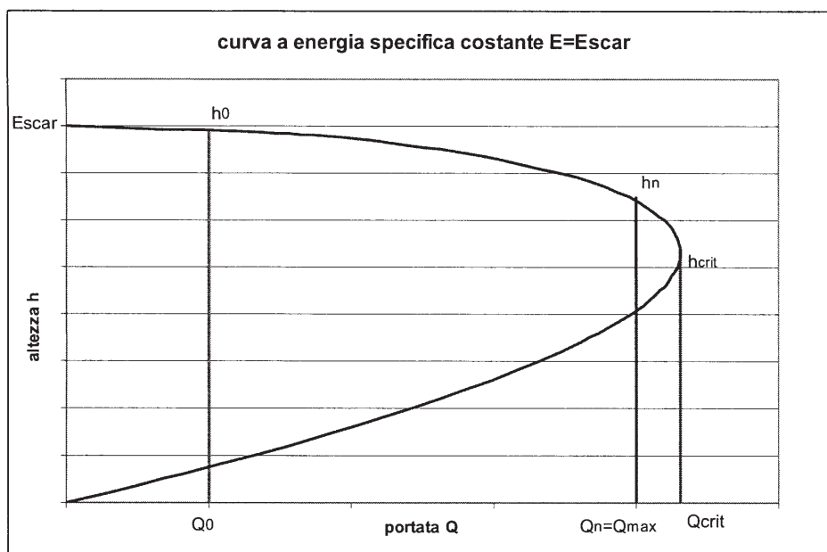
Figura 7: Curva h=h(Q) ad energia specifica costante /13/
